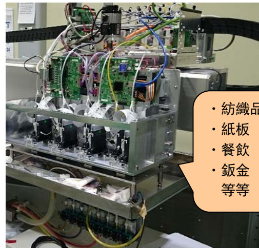
1800mm 紡織品 彩色印刷裝置頂部
